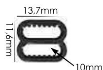
Ref.: APR 007 10mm Espessura: 1,7mm Materiais: POM, PP e PC Embalagem: 1000 unidades
