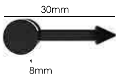
Ref.: APP 001 30x8mm Espessura: 2,3mm Materiais: POM e PC Embalagem: 1000 unidades
