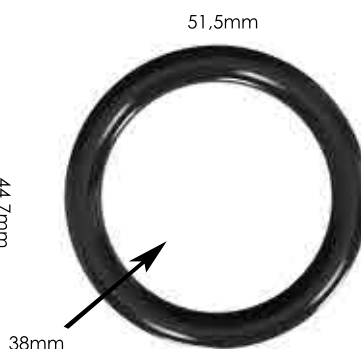
Ref.: APA 015 38mm Espessura: 5,2mm Materiais: PS Embalagem: 48 unidades
