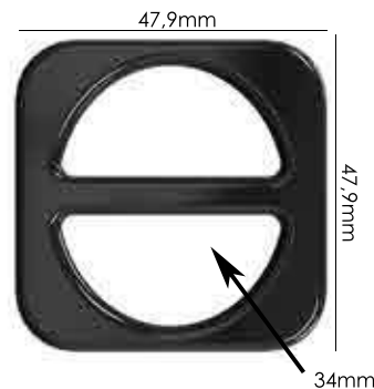
Ref.: APQ 001 34mm Espessura: 3,9mm Materiais: POM, PC e HS Embalagem: 100 unidades
