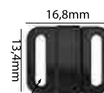
Ref.: APF 006 10mm Espessura: 4,5mm Materiais: POM, PC e HS Embalagem: 1000 unidades
