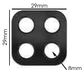
Ref.: APQ 4F 8mm Espessura: 2,1mm Materiais: POM e PC Embalagem: 200 unidades
