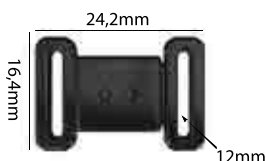
Ref.: APF 017 12mm Espessura: 3,2mm Materiais: POM, PC e HS Embalagem: 1000 unidades
