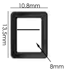
Ref.: APQ 003 8mm Espessura: 1,3mm Materiais: POM, PC e HS Embalagem: 1000 unidades
