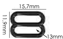
Ref.: APR 003/B 13mm Espessura: 1,4mm Materiais: POM, PP, PC e HS Embalagem: 1000 unidades
