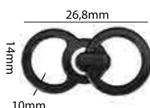
Ref.: APF 013 10mm Espessura: 1,3mm Materiais: POM, PC e HS Embalagem: 1000 unidades
