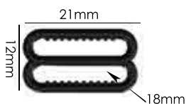
Ref.: APR 014 18mm Espessura: 2mm Materiais: POM, PC e HS Embalagem: 1000 unidades
