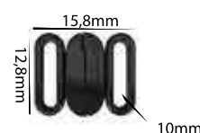
Ref.: APF 019 10mm Espessura: 2,5mm Materiais: POM, PC e HS Embalagem: 1000 unidades
