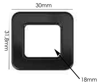
Ref.: APQ 002 18mm Espessura: 2,6mm Materiais: POM, PC e HS Embalagem: 200 unidades
