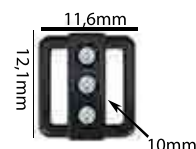
Ref.: APR 001 8 e 10mm Espessura: 2,6mm Materiais: POM e PC Acabamentos: Cristal ou Oktant Swarovski Embalagem: 100 unidades
