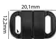
Ref.: APF 002 8mm Espessura: 3,6mm Materiais: POM, PC e HS Embalagem: 500 unidades
