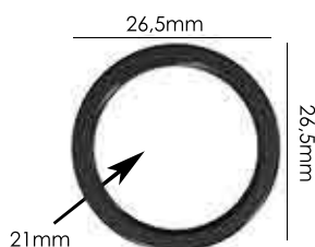
Ref.: APA 012 21mm Espessura: 2mm Materiais: POM Embalagem: 500 unidades
