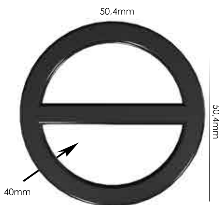
Ref.: APA PARALELA C/ TRAV 40MM Espessura: 2,4mm Materiais: POM, PC e HS Embalagem: 200 unidades
