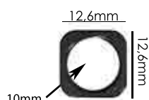
Ref.: APA 001/B 10mm Espessura: 1,4mm Materiais: POM, PP, PC e HS Embalagem: 1000 unidades
