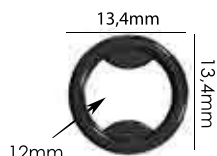
Ref.: APA 002 12mm Espessura: 1,4mm Materiais: POM, PP, PC e HS Embalagem: 1000 unidades
