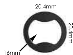
Ref.: APA 011 PARALELA 16mm Espessura: 1,5mm Materiais: POM, PP e PC Embalagem: 1000 unidades
