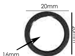
Ref.: APA 008 16mm Espessura: 1,6mm Materiais: POM, PC e HS Embalagem: 1000 unidades
