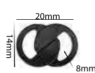
Ref.: APF 015 8mm Espessura: 2,4mm Materiais: POM, PC e HS Embalagem: 1000 unidades
