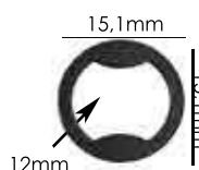
Ref.: APA 010 PARALELA 12mm Espessura: 1,3mm Materiais: POM Embalagem: 1000 unidades
