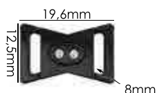
Ref.: APF 005 8mm Espessura: 2,8mm Materiais: POM e PC Acabamentos: Cristal ou Oktant Swarovski Embalagem: 100 unidades
